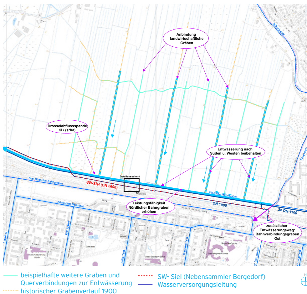
Entwässerungskonzept, 2017
